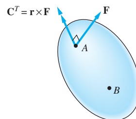
(b) Sistema equivalente fuerza-par
