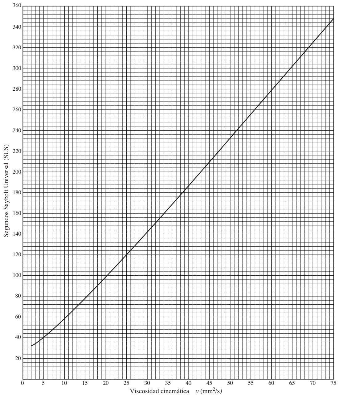
FIGURA 2.12 Viscosidad cinemática v expresada en SUS versus la expresada en mm 2 /s a 100 °F.
