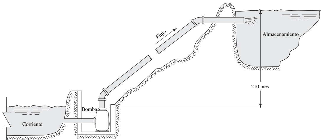
FIGURA 8.18 Problemas 8.46 y 8.47.
