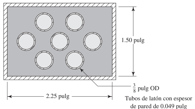
FIGURA 9.25 Problema 9.47.
