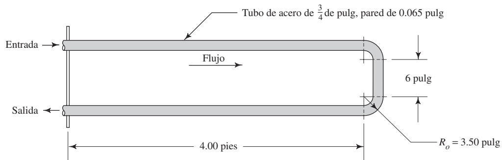
FIGURA 10.32 Problema 10.38.
