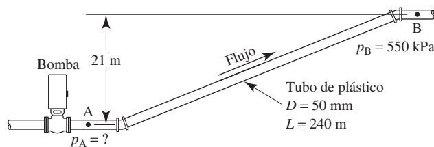
FIGURA 8.8 Problema modelo 8.8.
