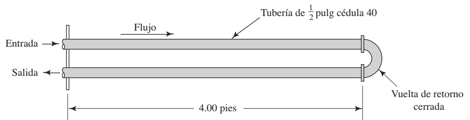
FIGURA 10.31 Problema 10.37.
