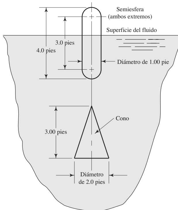
FIGURA 5.22 Problema 5.16.
