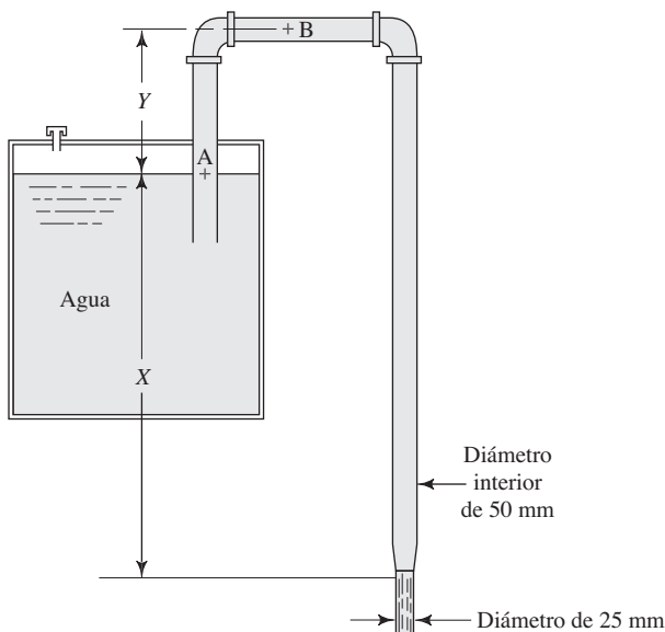
FIGURA 6.25 Problemas 6.69, 6.70 y 6.71.
