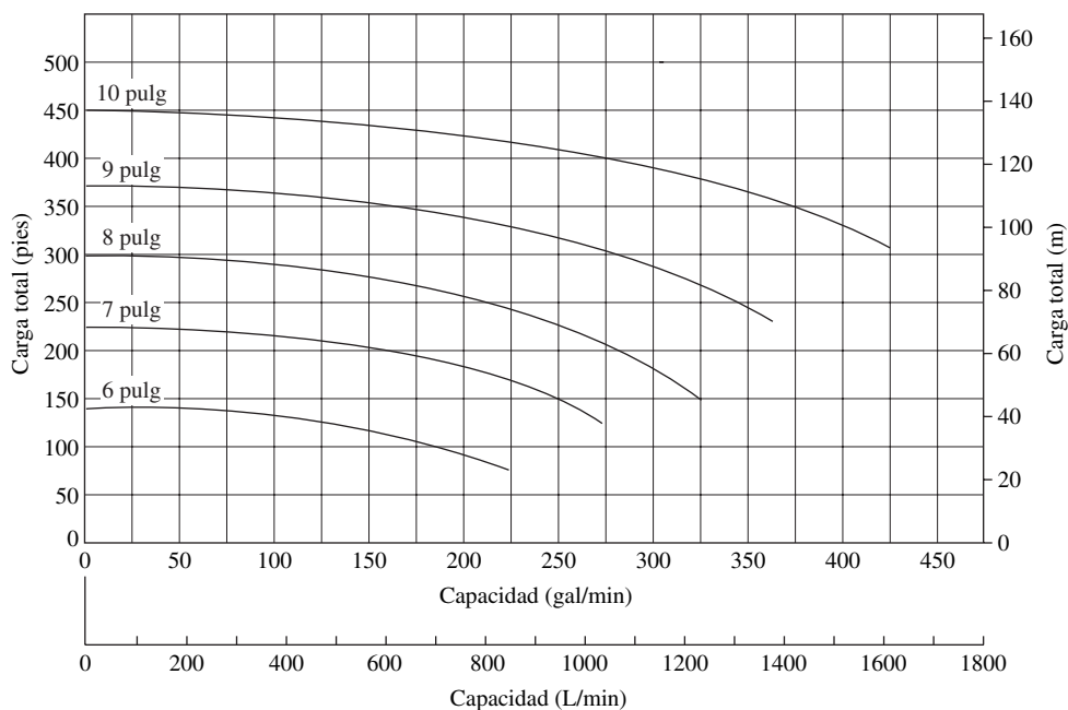
FIGURA 13.22 Ilustración del rendimiento de una bomba para diámetros diferentes del impulsor. Gráfica de rendimiento de una bomba centrífuga de 2 \times 3 - 10 , a 3500 rpm.
