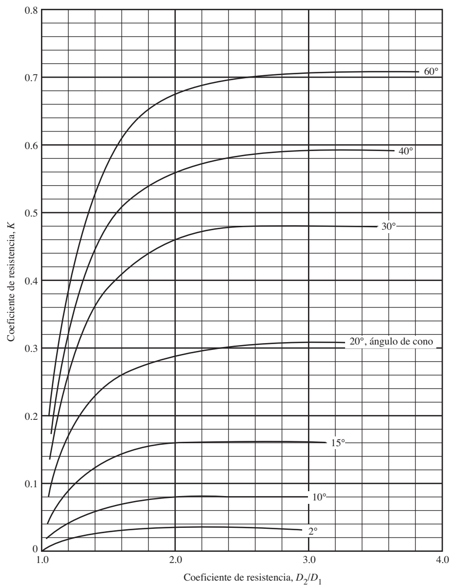
FIGURA 10.5 Coeficiente de resistencia-expansión gradual.
