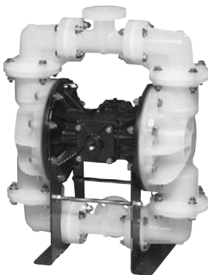
(a) Bomba de diafragma con carcasa no metálica
