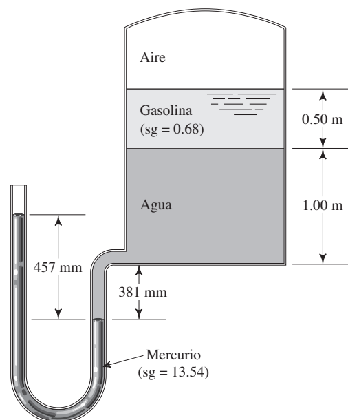
FIGURA 3.24 Problema 3.54.
