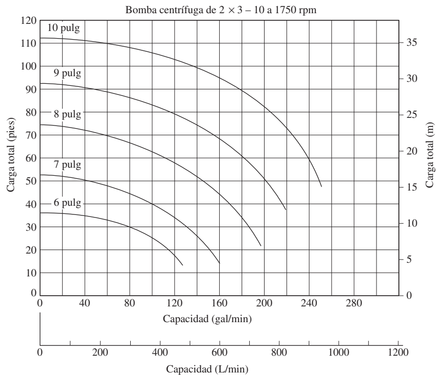
FIGURA 13.23 Rendimiento de una bomba centrífuga de 2 \times 3 - 10 , cuando opera a 1750 rpm.
