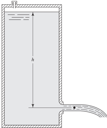
FIGURA 6.37 Tanque para los problemas 6.87 y 6.88.
