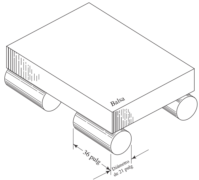
FIGURA 5.27 Problemas 5.31, 5.33 y 5.34.
