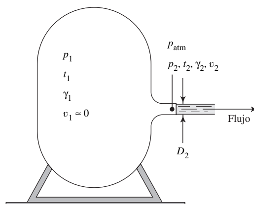
FIGURA 18.10 Descarga de un gas de un tanque a través de una boquilla lisa y convergente.
