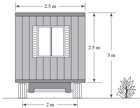
FIGURA 17.13 Problema 17.12.
