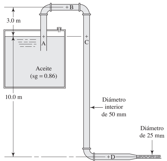
FIGURA 6.26 Problema 6.72 y 6.83.
