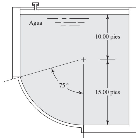
FIGURA 4.49 Problema 4.49.
