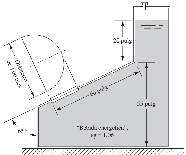
FIGURA 4.56 Problema 4.64.
