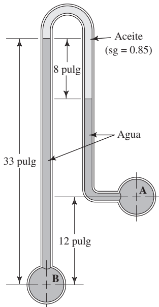
FIGURA 3.29 Problema 3.64.
