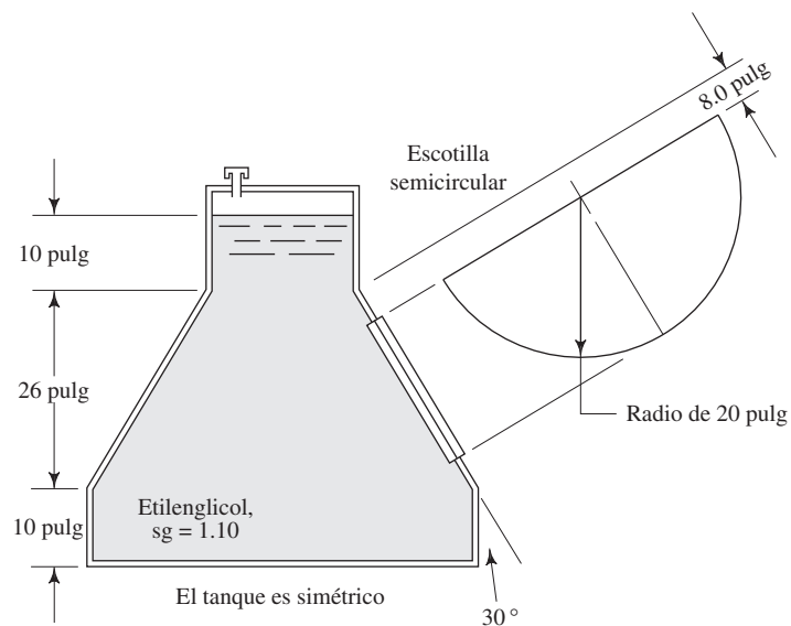
FIGURA 4.40 Problemas 4.28 y 4.46.
