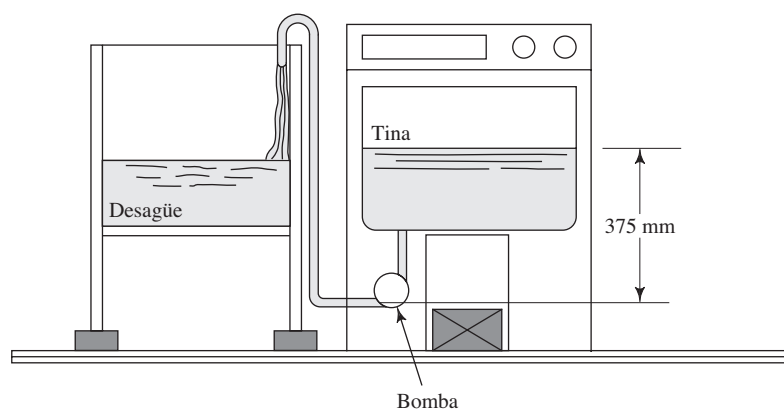
FIGURA 3.21 Máquina lavadora de ropa del problema 3.42.
