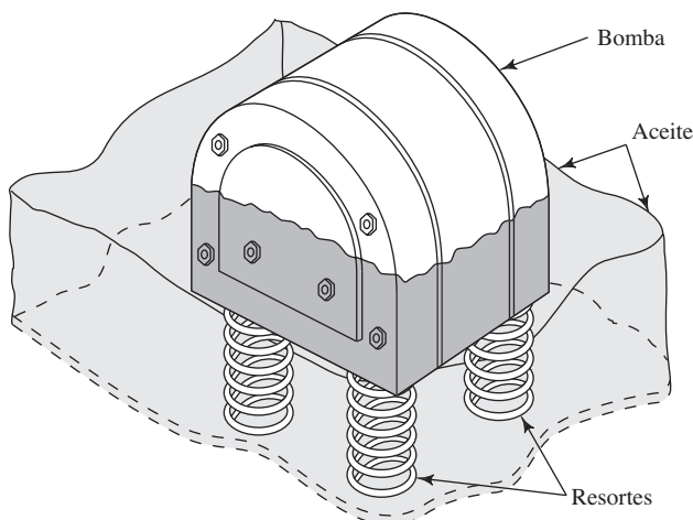
FIGURA 5.19 Problema 5.8.
