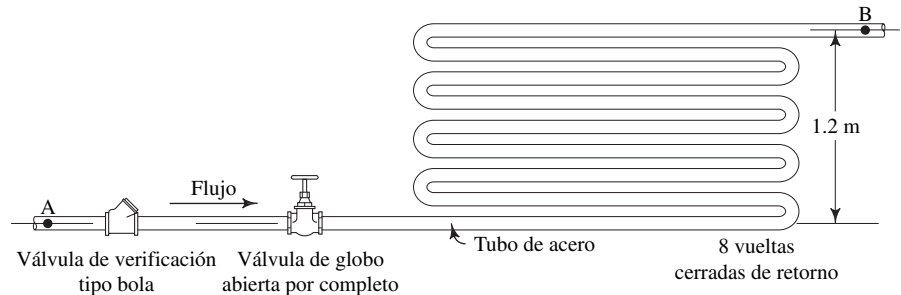
FIGURA 11.17 Problema 11.7.
