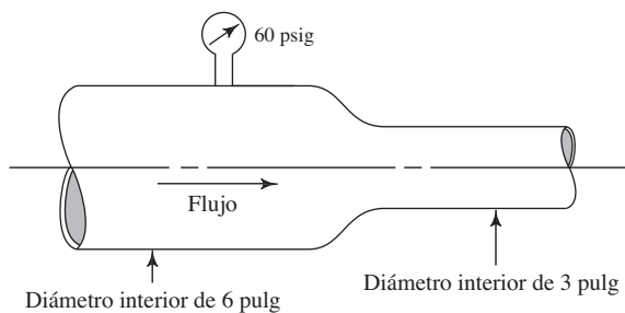
FIGURA 6.33 Problema 6.81.
