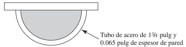
FIGURA 9.29 Problema 9.51.
