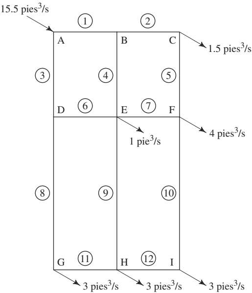
FIGURA 12.13 Problema 12.11.
