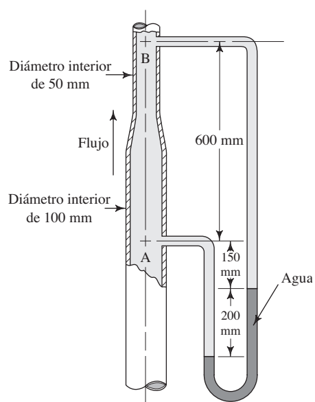
FIGURA 6.30 Problema 6.77.
