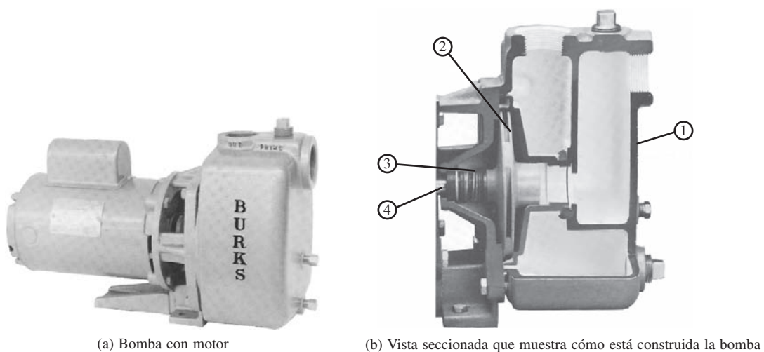
FIGURA 13.16 Bomba de autoarranque. (1) Carcasa de la entrada de succión, (2) impulsor, (3) sello del eje mecánico, (4) eje. (Fuente: Crane Pumps & Systems, Piqua, OH.)
