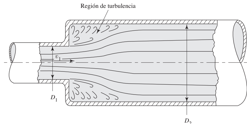
FIGURA 10.1 Expansión súbita.
