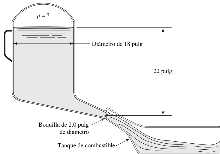
FIGURA 7.37 Problema 7.41.
