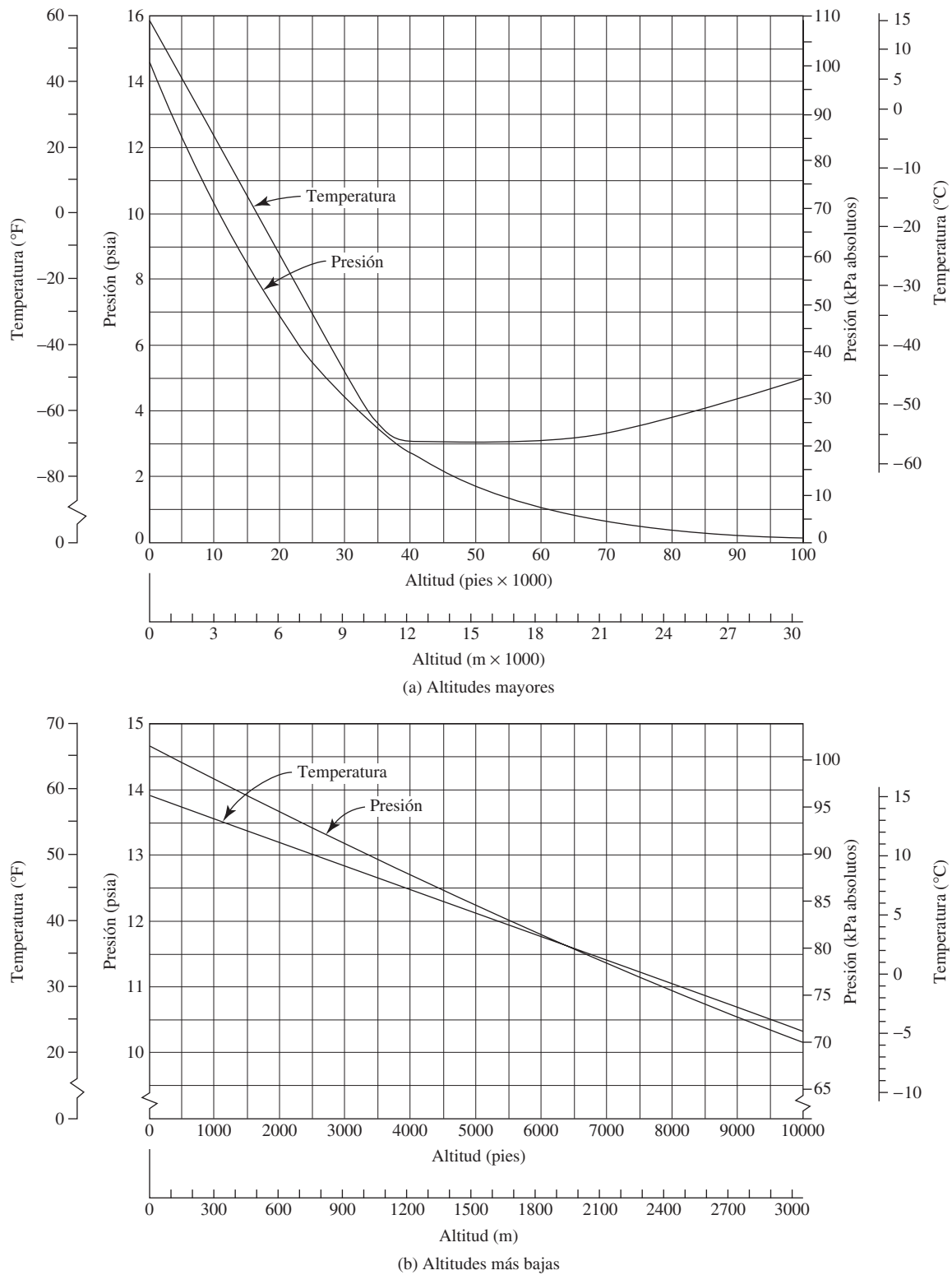
FIGURA E.1 Propiedades de la atmósfera estándar versus la altitud.
