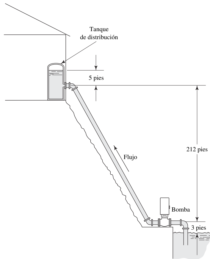
FIGURA 7.38 Problemas 7.42 y 7.43.
