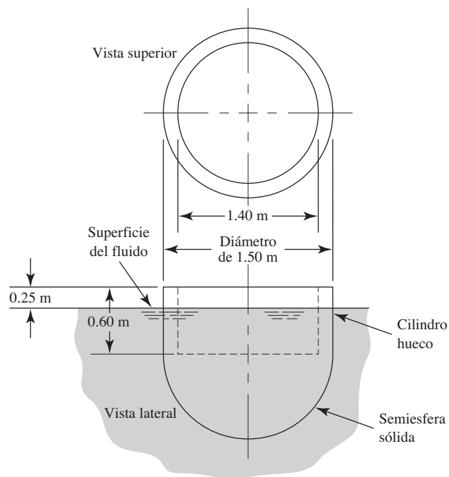
FIGURA 5.35 Problema 5.63.
