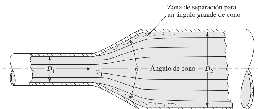
FIGURA 10.4 Expansión gradual.
