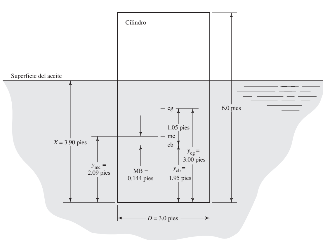
FIGURA 5.15 Solución completa para el problema modelo 5.6.
