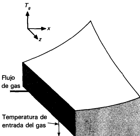
Fig. 10-6 Perfil típico de temperatura para el cambiador de calor de flujo transversal de la Fig. 10-5.
