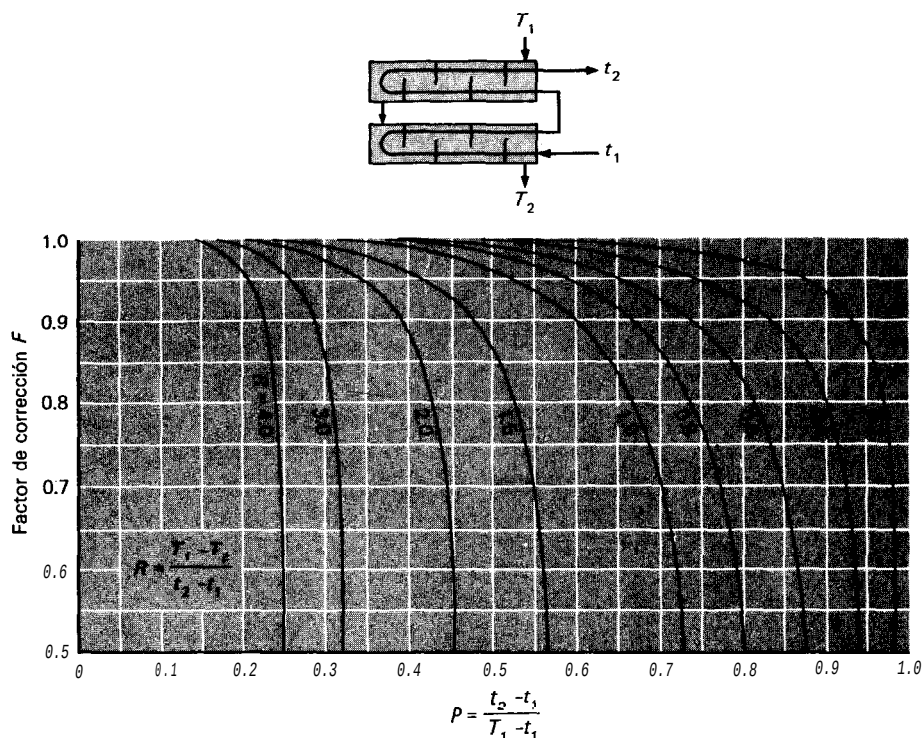
Fig. 10-9 Diagrama del factor de corrección para un cambiador de calor con dos pasos en la chaqueta y cuatro, ocho o cualquier otro múltiplo de pasos en los tubos.
