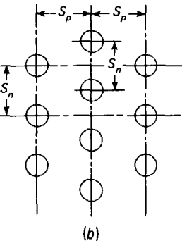
Fig. 6-14 Nomenclatura que se utiliza con la Tabla 6-4: (a) hileras alineadas; (b) hileras de tubos alternadas.
