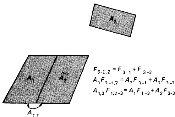
Fig. 8-19 Esquema que muestra algunas relaciones entre los factores de forma.
