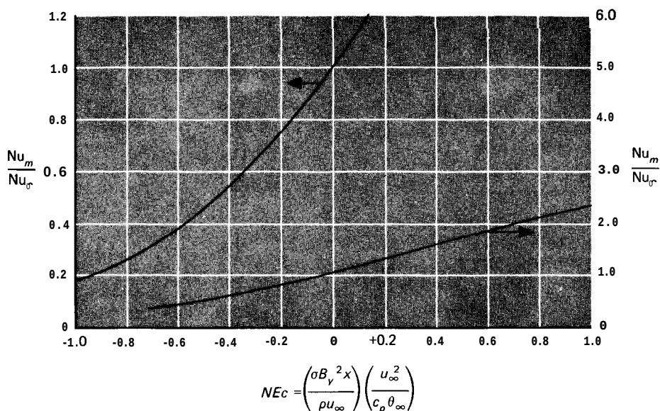
Fig. 12-4 Influencia del campo magnético en la transferencia de calor en una placa plana.
