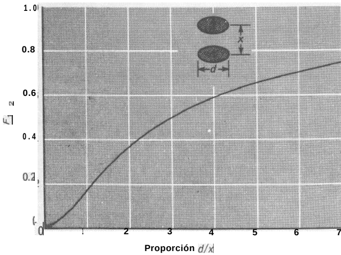
Fig. 8-13 Factor de forma de la radiación para radiaciones entre discos paralelos.
