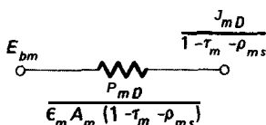
Fig. 8-59 Elemento de red que representa la Ec. 8-93.
