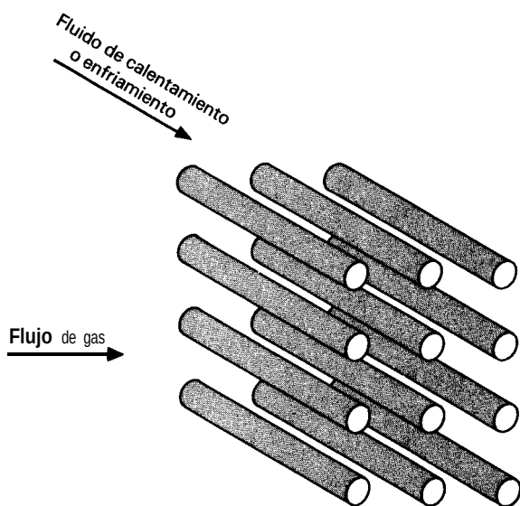
Fig. 10-4 Cambiador de calor de flujo transversal con un fluido mezclado y otro sin mezclar.
