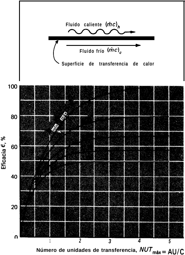
Fig. 10-12 Eficacia para el rendimiento de un cambiador de flujo paralelo.
