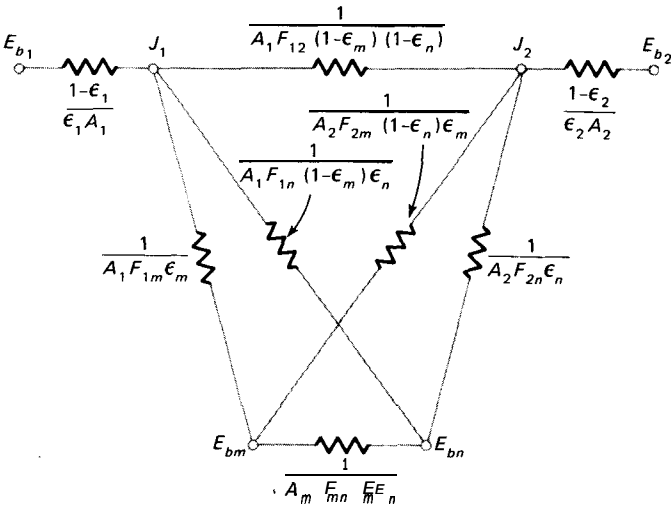
Fig. 8-47 Red total de radiación para el sistema de la Fig. 8-43.
