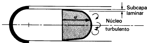
Rg. 815 Perfil de velocidad en flujo turbulento en tubos.
