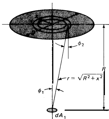
Fig. g-II Radiación de un pequeño elemento de área hacia un disco.
