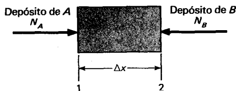
Fig. 11-3 Esquema que ilustra difusión equimolal.
