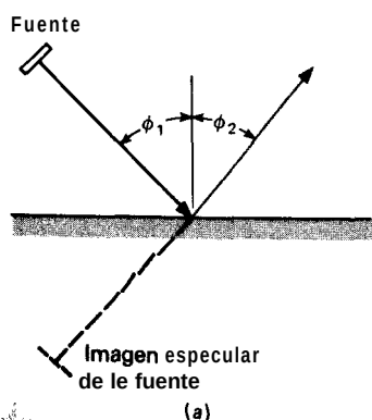
Fig. 8-3 Reflexiones (a) especular ( \phi_1 = \phi_2 ) y (b) difusa.
