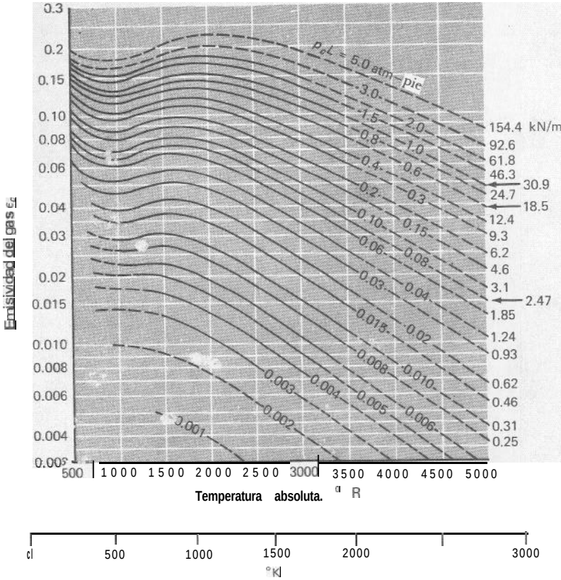
Fig. 8-34 Emisividad para bióxido de carbono, para una presión total = 1 atm; 1.0 kN/m = 0.03238 atm·pie, de acuerdo con la Ref. 22.
