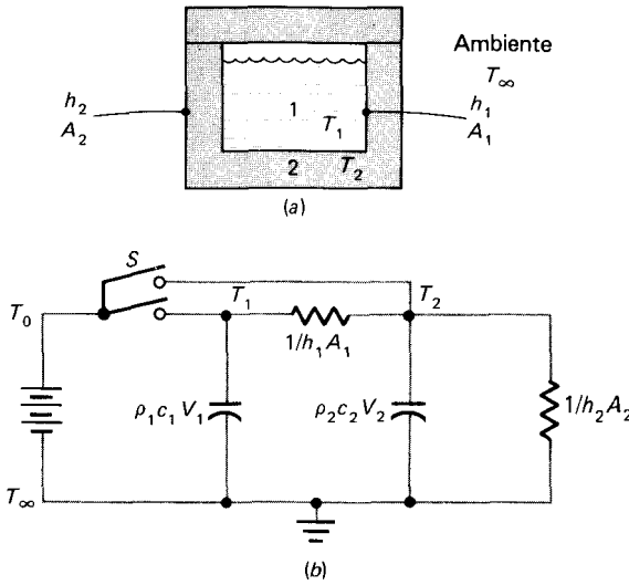
Fig. 43 Nomenclatura para análisis de capacidad calorífica en dos partes.
