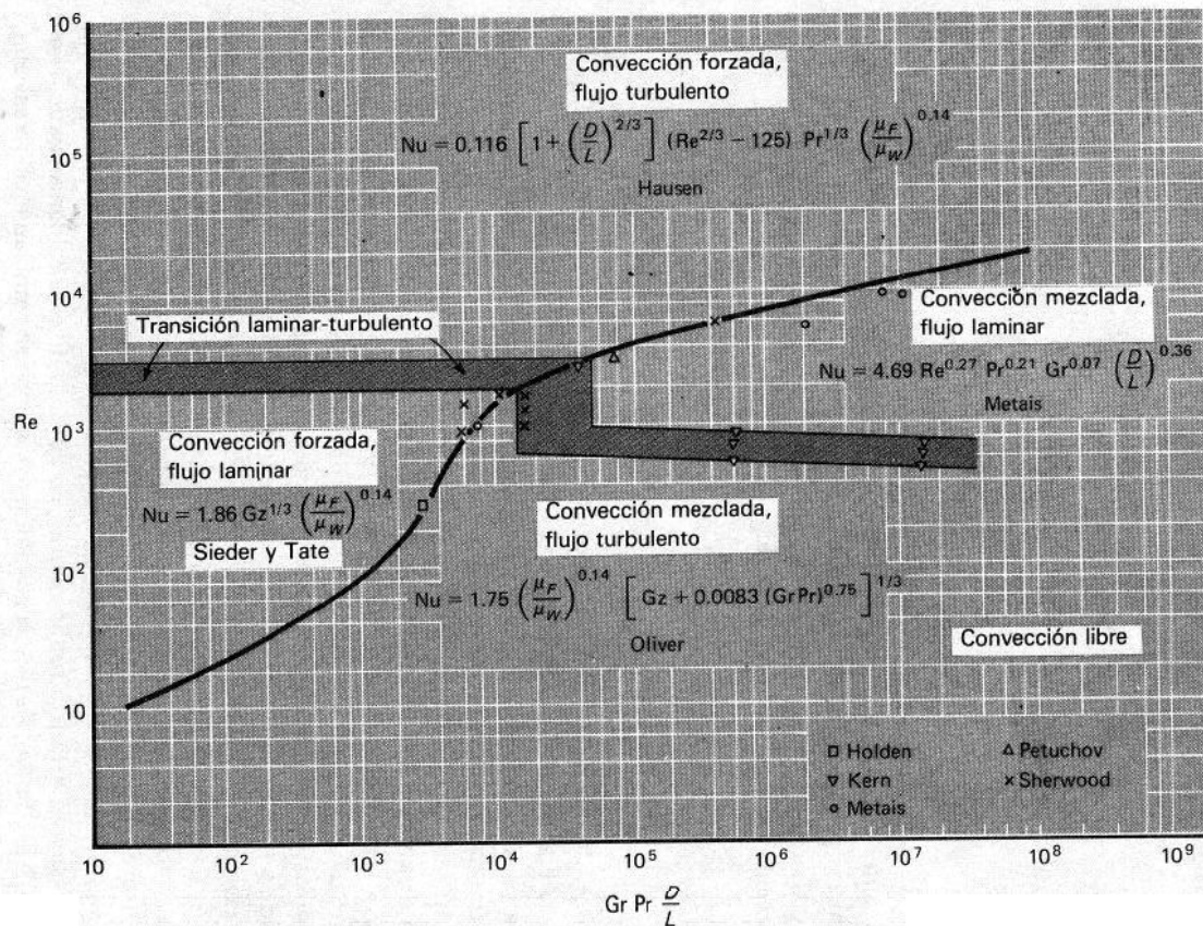
Fig. 7-14 Régimenes de convección libre, forzada y mezclada para flujo a través de tubos horizontales, de acuerdo con Metais y Eckert [10]
