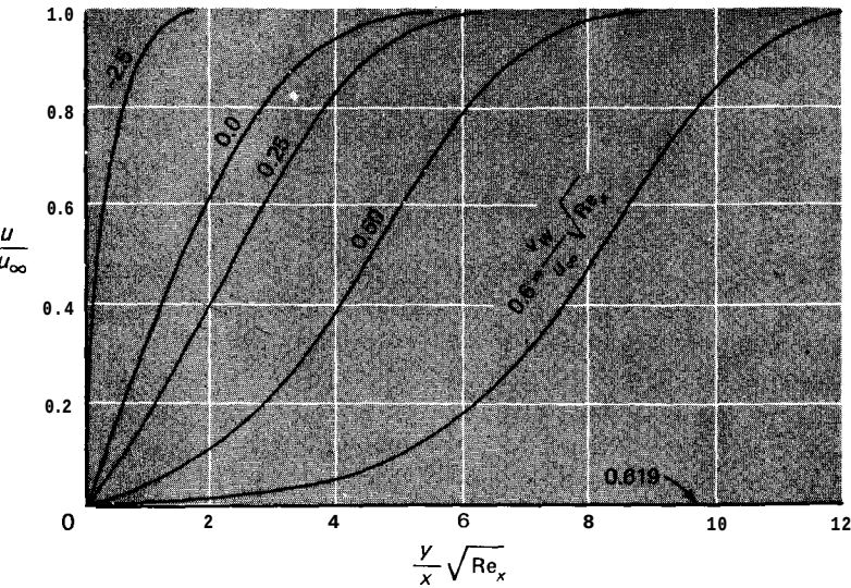
Fig. 12-6 Perfiles de velocidad en capa límite laminar para inyección en una placa plana, según la Ref. 3.
