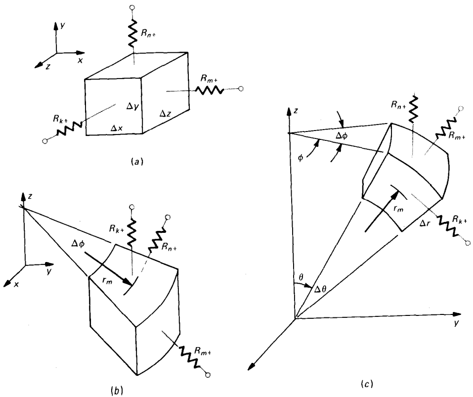
Fig. 3-11 Elementos de volumen y resistencia: Sistemas coordenados (a) cartesiano, (b) cilíndrico y (c) esférico.
