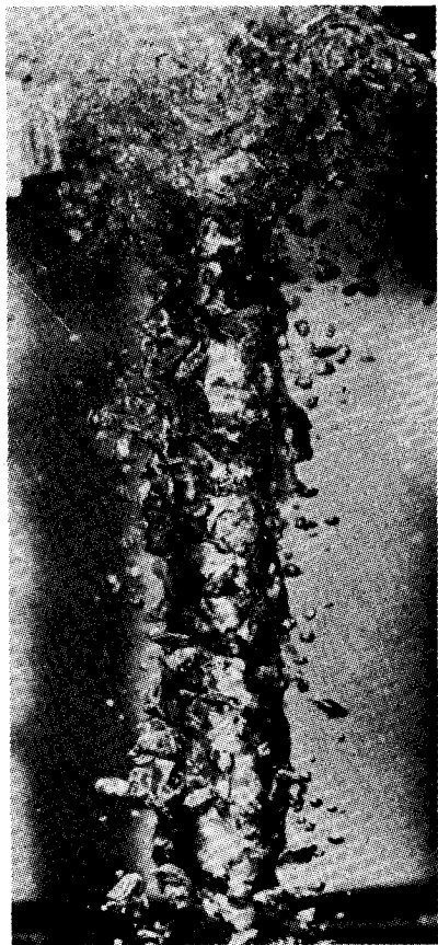
Fig. 9-6 Ebullición por película turbulenta de metanol en un tubo vertical de cobre de 19.05 mm de diámetro, calentado por vapor, de la Ref. 41; q/A = 38.8 \text{ kW/m}^2 , \Delta T_s = 138^\circ \text{C} . (Fotografías por cortesía del Prof. J. W. Westwater.)
