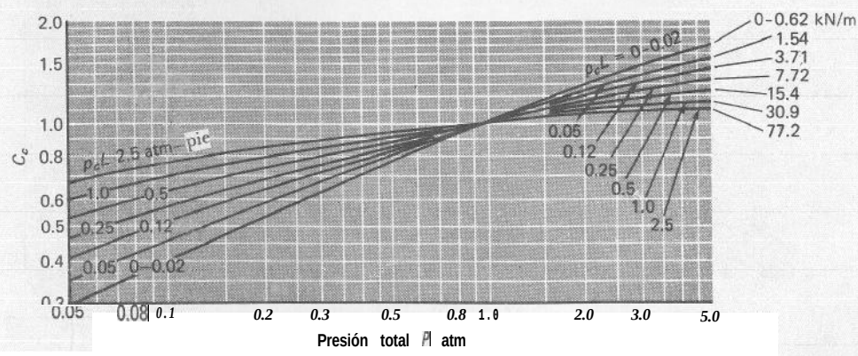
Fig. 8-36 Factor de corrección para emisividad de CO, de acuerdo con la Ref. 22.
