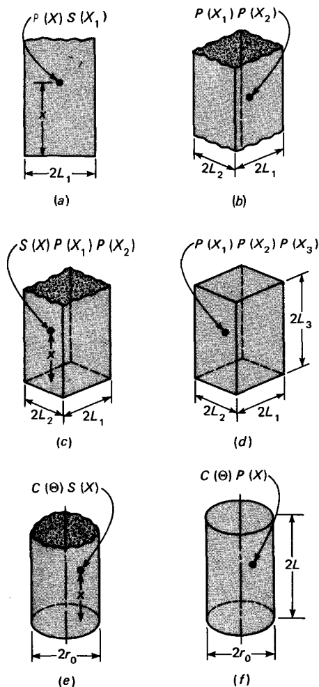
Fig. 4-20 Soluciones de producto para temperaturas en sistemas multidimensionales: (a) placa semiinfinita; (b) barra rectangular infinita; (c) barra rectangular semiinfinita; (d) paralelepípedo rectangular; (e) cilindro semiinfinito; (f) cilindro corto.
