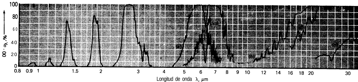
Fig. 8-33 Absorbencia monocromática del vapor de agua de acuerdo con la Ref. 8. Para longitudes de onda de 0.8 a 4 \mu\text{m} , temperatura del vapor 127 °C, espesor de capa 109 cm; longitudes de onda de 4 a 34 \mu\text{m} ; (a) temperatura 127 °C, espesor de capa 109 cm; (b) temperatura 127 °C, espesor de capa 104 cm; (c) temperatura 127 °C, espesor de capa 32.4 cm; (d) temperatura 81 °C, espesor de capa 32.4 cm, mezcla con corriente de aire correspondiente a una capa de vapor de espesor aproximado de 4 cm; (e) temperatura ambiente, capa de aire húmedo de 200 cm de espesor correspondiente a una capa de vapor a presión atmosférica de espesor aproximado de 7 cm.
