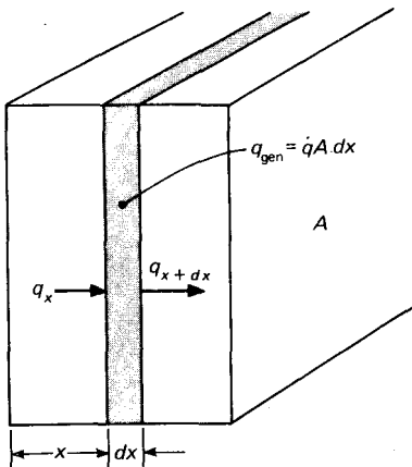
Fig. 1-2 Volumen elemental para el análisis de la conducción de calor unidimensional.
