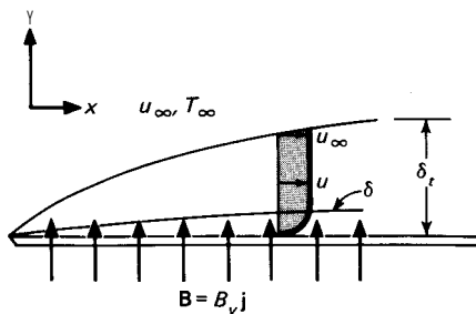
Fig. 12-3 Capa límite térmica en flujo de dinámica de magnetofluido.
