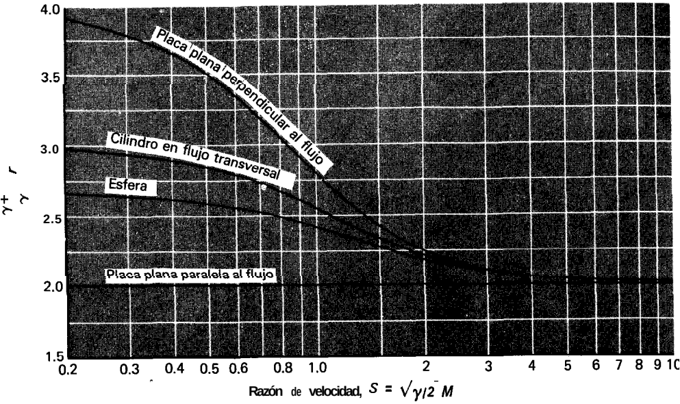
Fig. 12-16 Factores de recuperación para flujo molecular libre, de acuerdo con la Ref. 8.
