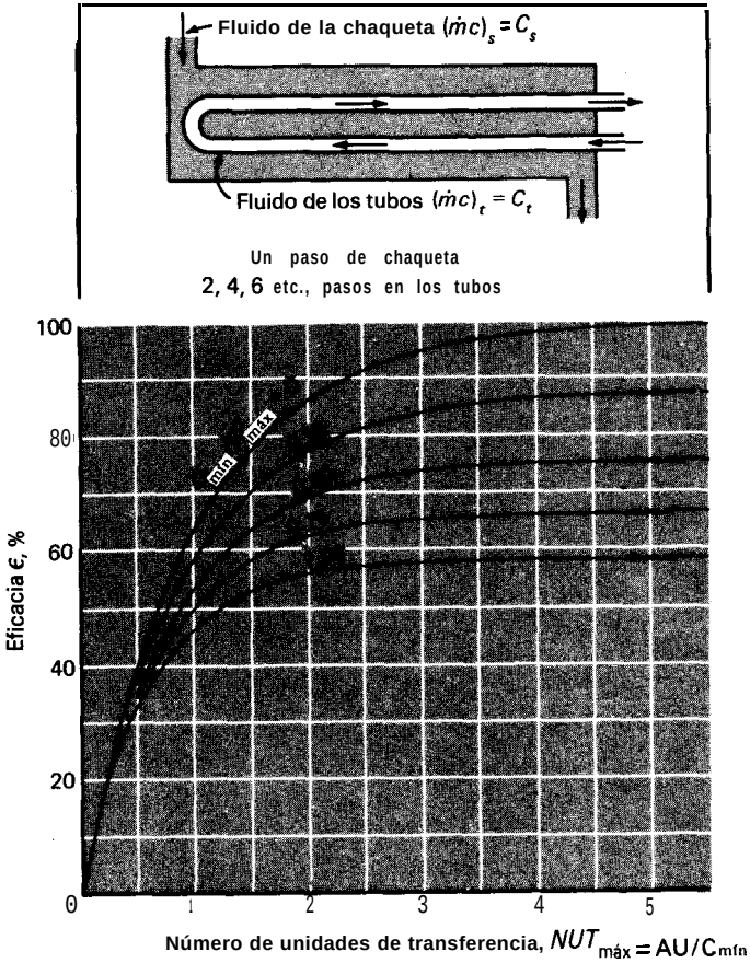
Fig. 10-16 Eficacia para el rendimiento de un cambiador de flujo a contracorriente paralelo 1-2.
