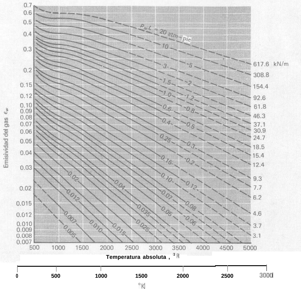
Fig. 8-35 Emisividad para el vapor de agua para presión total = 1 atm 1.0 kN/m = 0.03238 atm-pie de acuerdo con la Ref. 22.
