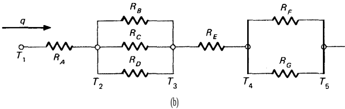
Fig. 2-2 Transferencia de calor unidimensional en serie o en paralelo a través de una pared compuesta y análogo eléctrico.
