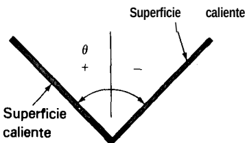
Fig. 7-9 Sistema de coordenadas para placas inclinadas.
