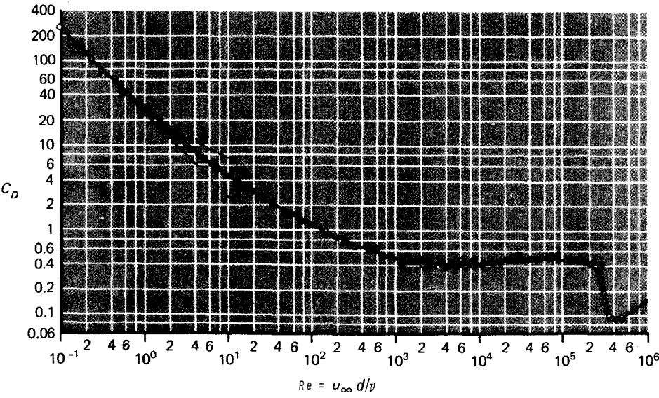
Fig. 6-10 Coeficiente de arrastre para esferas como una función del número de Reynolds, a partir de la Ref. 6.
