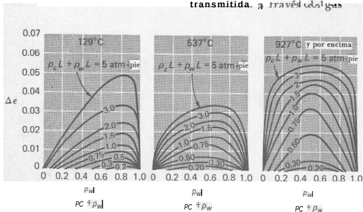
Fig. 8-38 Factor de corrección cuando están presentes \text{CO}_2 y \text{H}_2\text{O} en un recinto, de acuerdo con la Ref. 22: 1.0 atm-pie, = 30.881 kN/m
