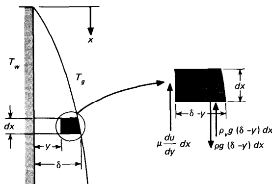
Fig. g-l Condensación por película en una placa plana vertical.
