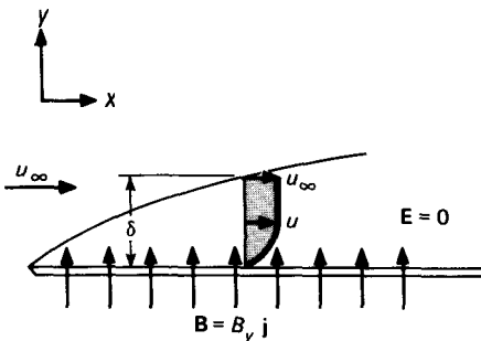
Fig. 12-1 Capa límite hidromagnética.
