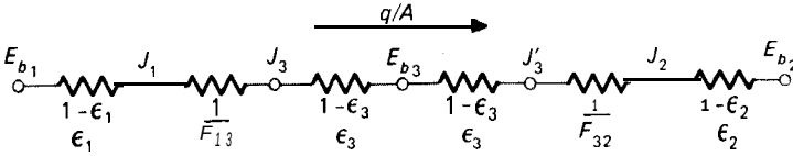
Fig. 8-31 Red de radiación para dos planos paralelos separados por una protección contra radiación.
