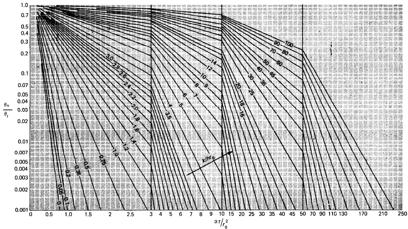
Fig. 4.11 Temperatura central para una esfera de radio r_0 , de la Ref. 2.
