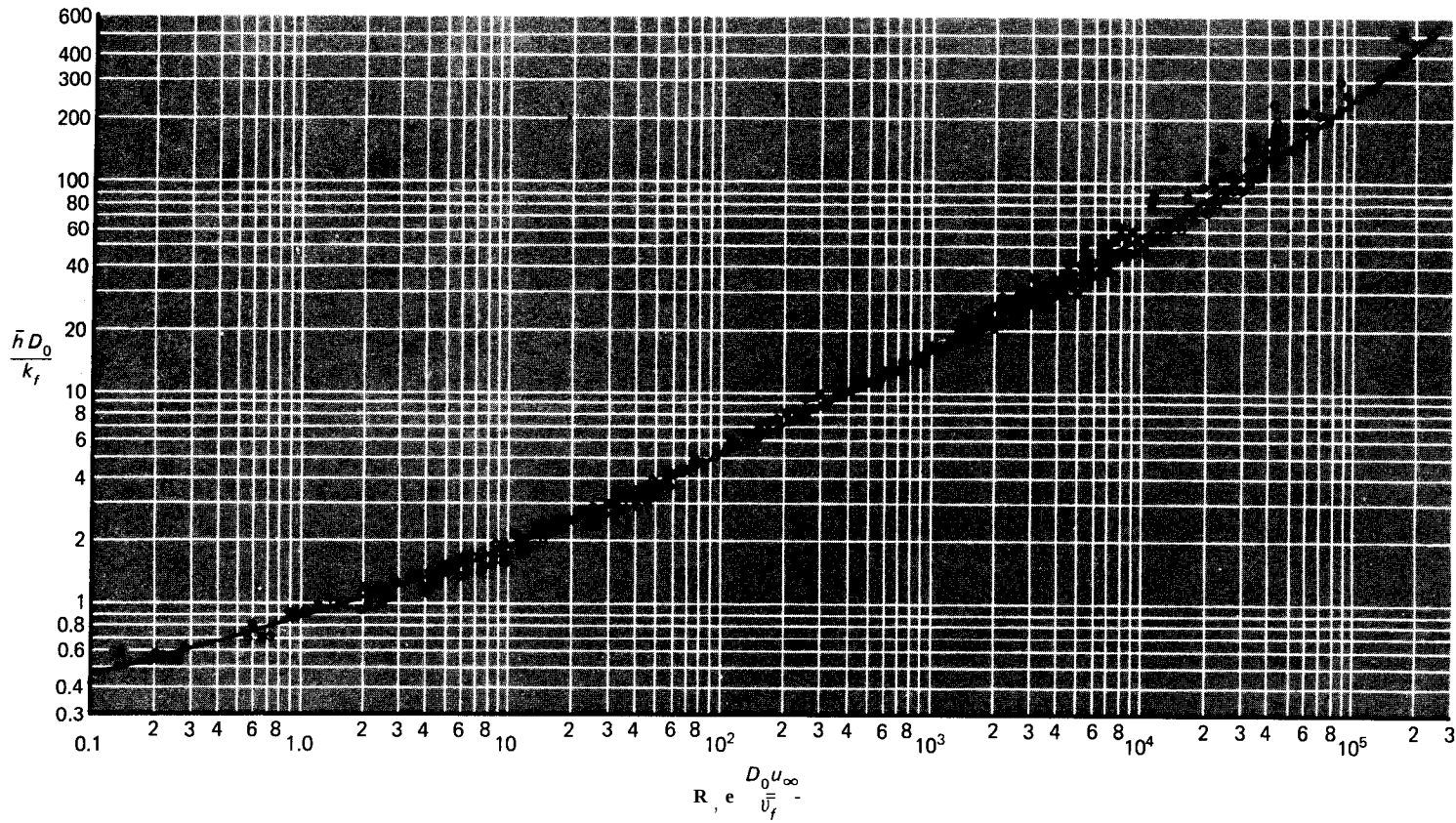
Fig. 6-12 Datos para calentamiento y enfriamiento de aire fluyendo normal a cilindros solos, de la Ref. 10.
