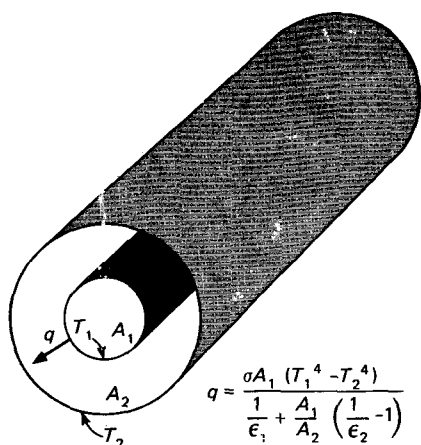
Fig. 8-29 Intercambio de radiación entre dos superficies cilíndricas.
