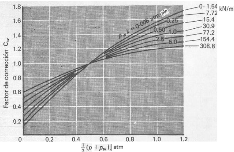
Fig. 8-37 Factor de corrección para emisividad de \text{H}_2\text{O} de acuerdo con la Ref. 22.
