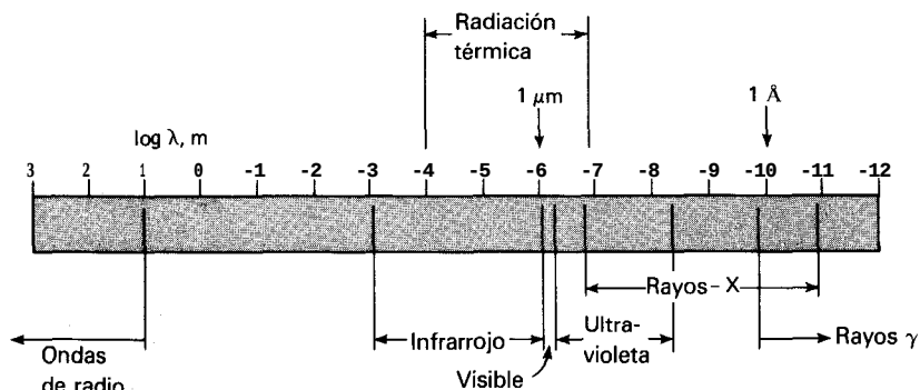
Fig. 8-1 Espectro electromagnético.
