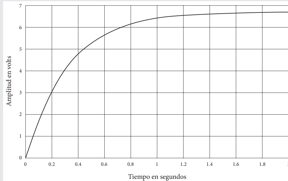
Figura 3.3 Gráfica del voltaje del capacitor.
