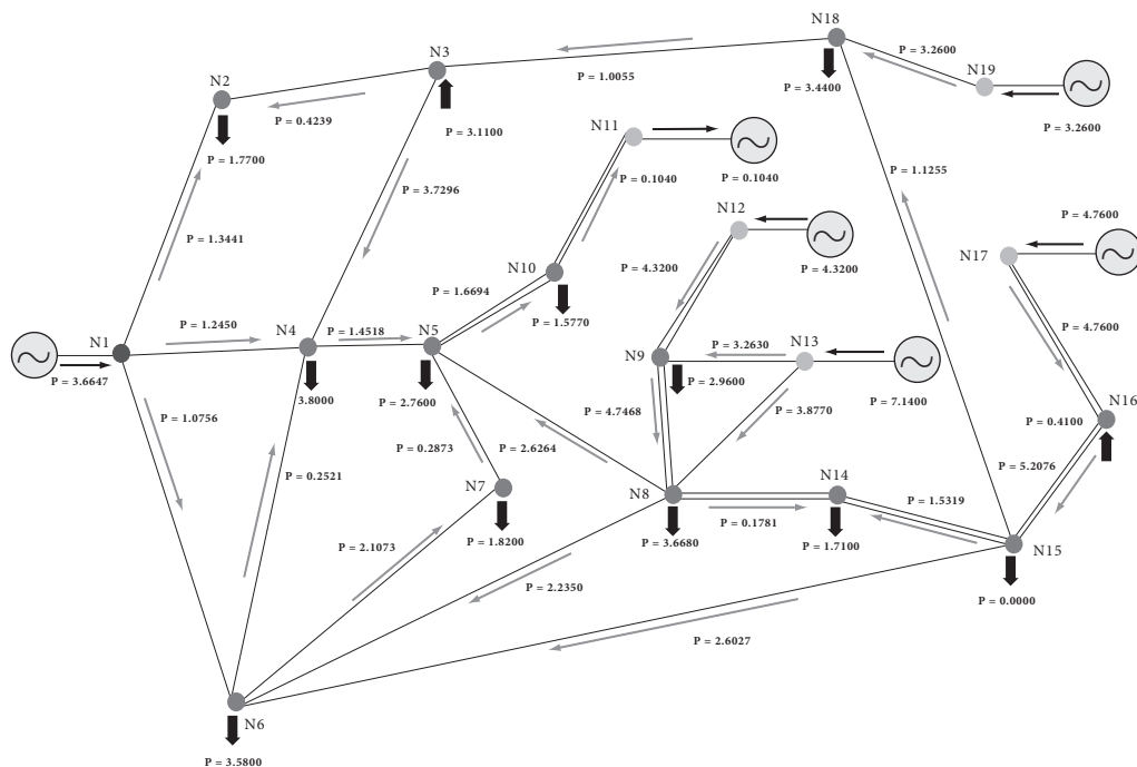
Figura 2.13 Flujo por cada línea.
