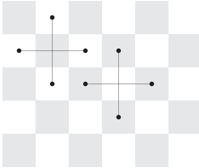
Figura 9.9 El origen de la inestabilidad es un esquema de salto de rana. Si tomamos a los puntos de la malla como cuadrados de un tablero de ajedrez, entonces los cuadrados blancos se acoplan entre sí, y los negros también; pero no hay acoplamiento entre negros y blancos. La estrategia aquí, es introducir una pequeña pieza de difusión que acople la malla.
