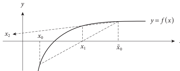
Figura 2.5 Divergencia del método de la secante.
