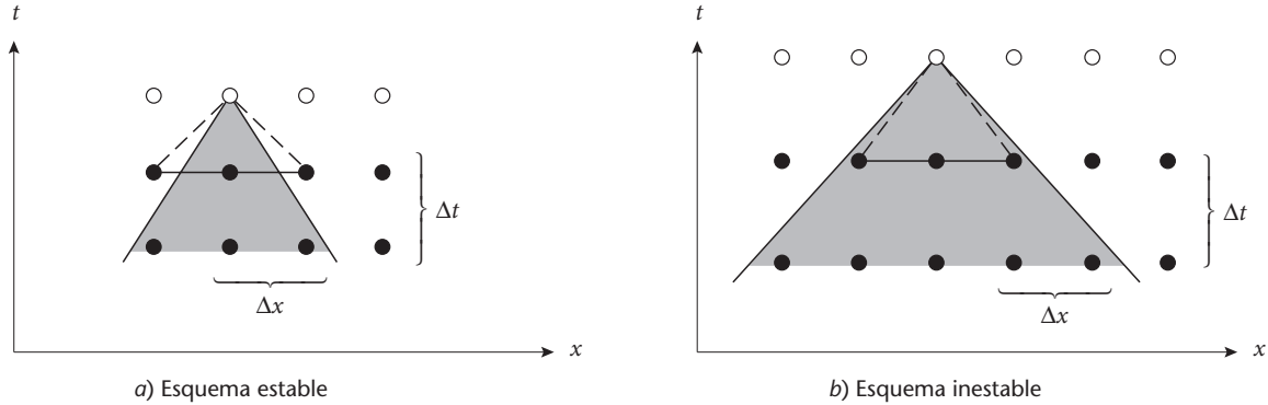
Figura 9.6 Condición de Courant para un esquema de diferenciación. Un esquema diferenciador de Courant es estable si el dominio de dependencia es más grande que el de la EDP, como en a); y es inestable si la relación es inversa, como b).
