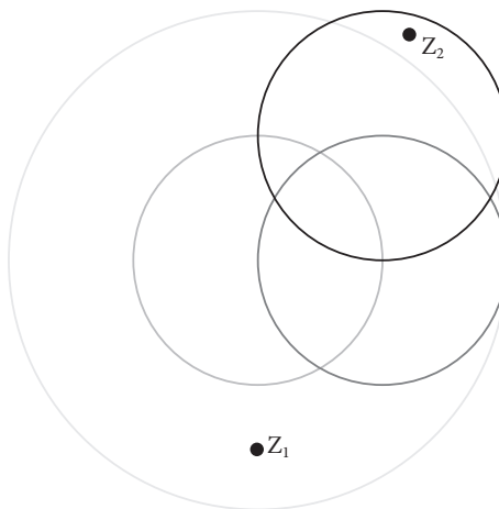
Figura 3.1 Método de Lehmer-Schur.
