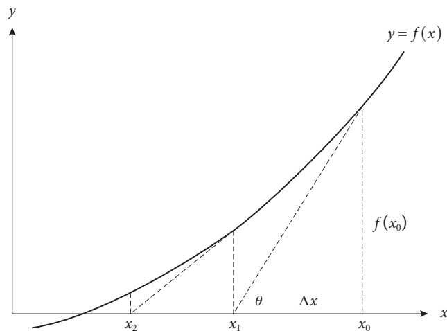
Figura 2.7 Método de Newton-Raphson.
