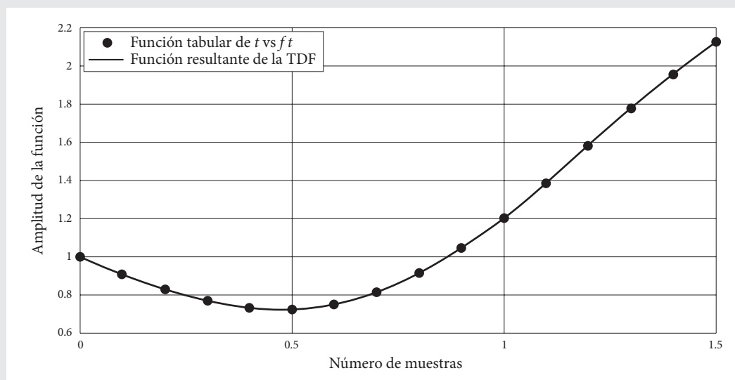
Figura 5.11 Descomposición discreta utilizando la TDF.
