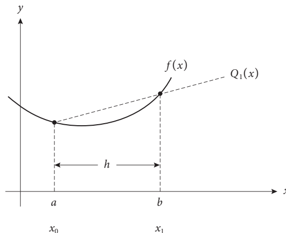
Figura 6.4 Gráfica de la regla trapezoidal.
