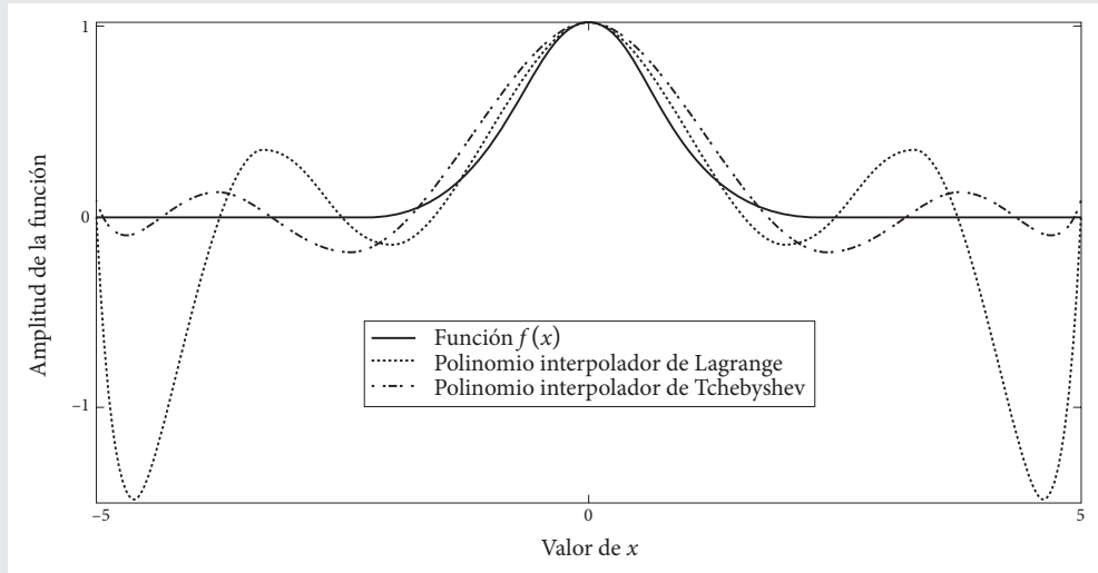
Figura 5.4 Gráfica de la función evaluada y de los dos polinomios interpoladores.
