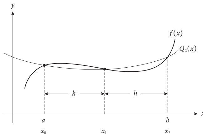
Figura 6.5 Gráfica de la regla de Simpson 1/3.
