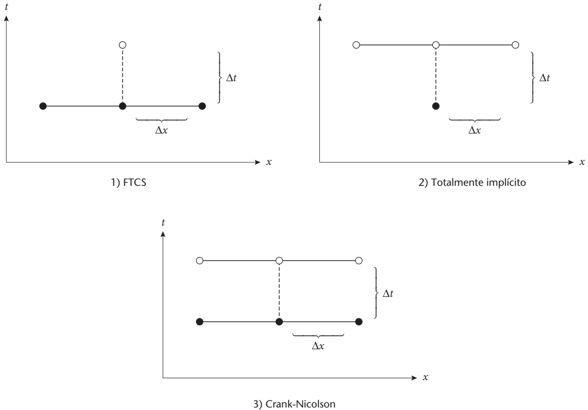
Figura 9.11 Tres esquemas de diferenciación para problemas de difusión.
