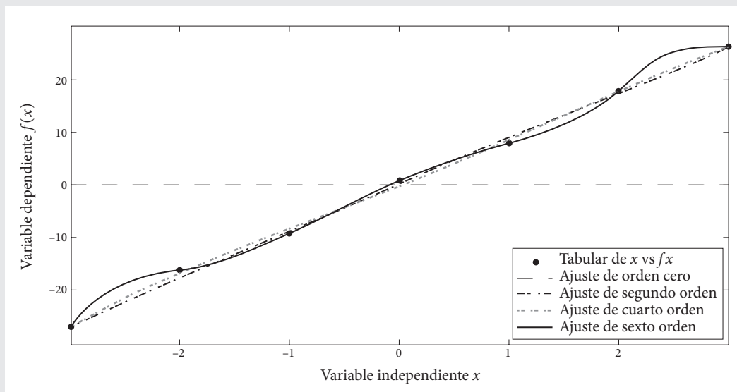
Figura 5.5 Gráfica de la tabla de datos y todas sus funciones de ajuste.
