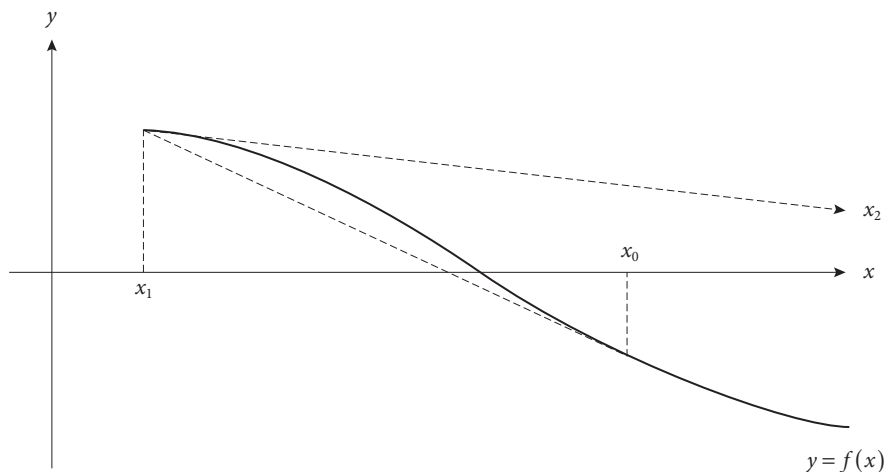
Figura 2.8 Divergencia del método de Newton-Raphson.
