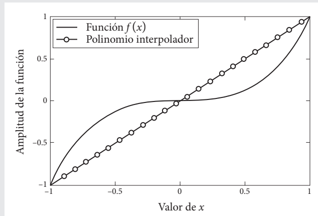
Figura 5.1 Gráfica de la función f(x) y del polinomio interpolador p(x) .
