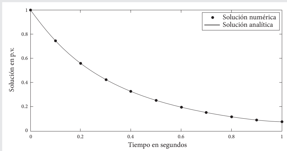
Figura 7.1 Solución numérica vs. solución analítica.
