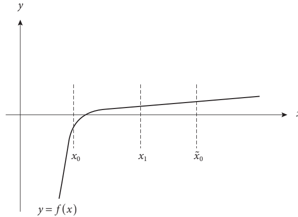
Figura 2.1 Método de bisección.
