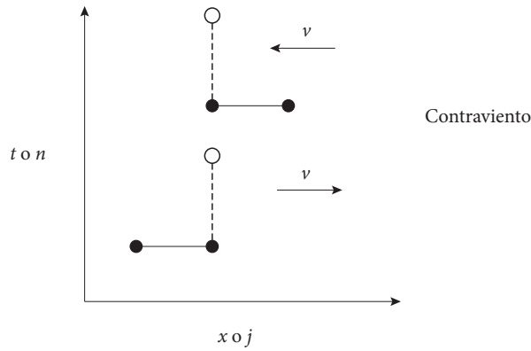
Figura 9.7 Representación de los esquemas diferenciadores contraviento. El esquema superior es estable cuando la constante de advección v es negativa, como se muestra. El esquema inferior es estable cuando la constante de advección es positiva.
