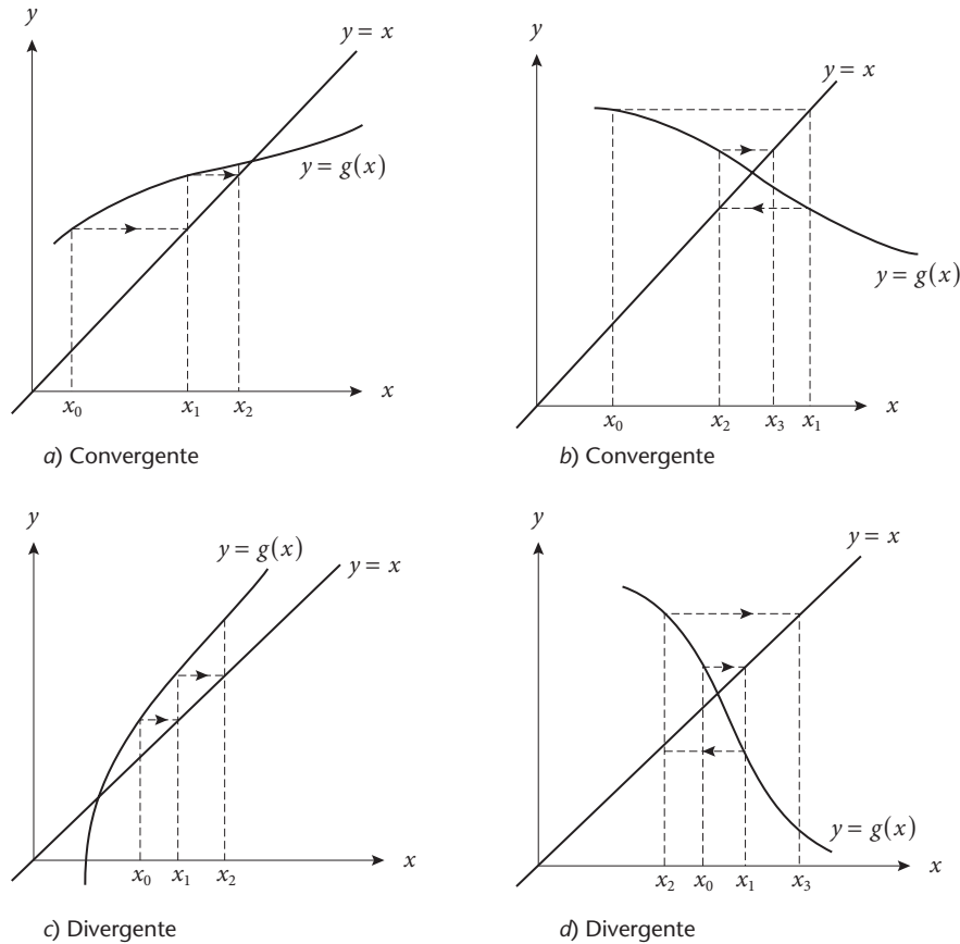
Figura 2.6 Método de punto fijo.
