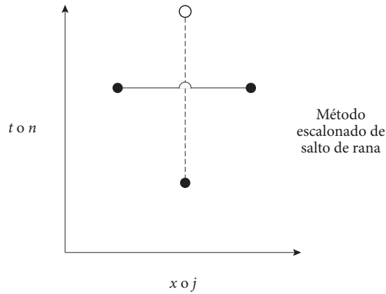
Figura 9.8 Representación del esquema diferenciador del salto de rana escalonado. Este esquema es muy preciso, de segundo orden en espacio y tiempo.
