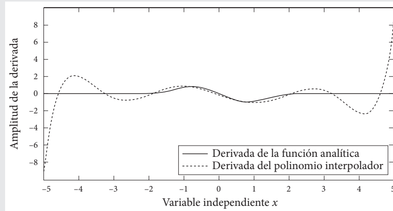
Figura 6.1 Gráfica de la derivada de la función evaluada y del polinomio interpolador.
