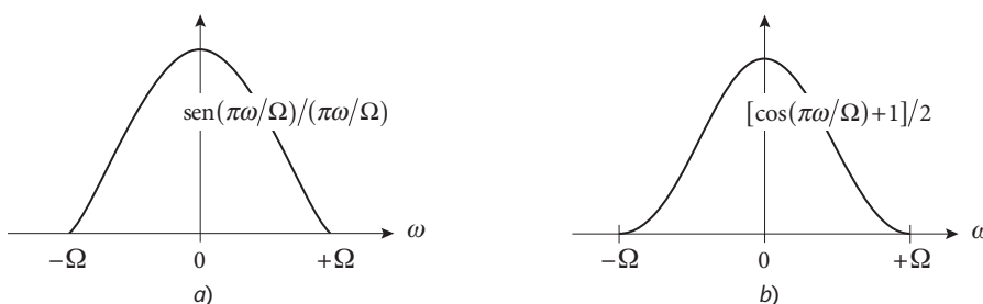
Figura 5.9 Ventana de datos a) Lanczos y b) Von Hann.
