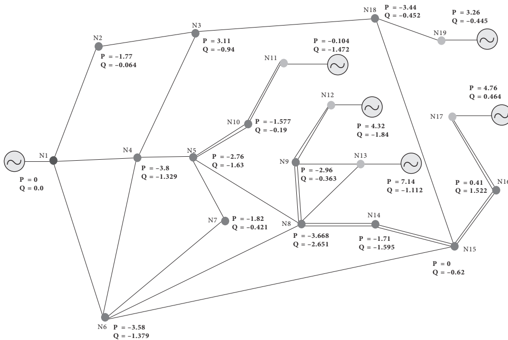
Figura 2.10 Datos de P y Q de la red trifásica.
