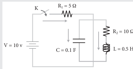
Figura 3.2 Circuito eléctrico.
