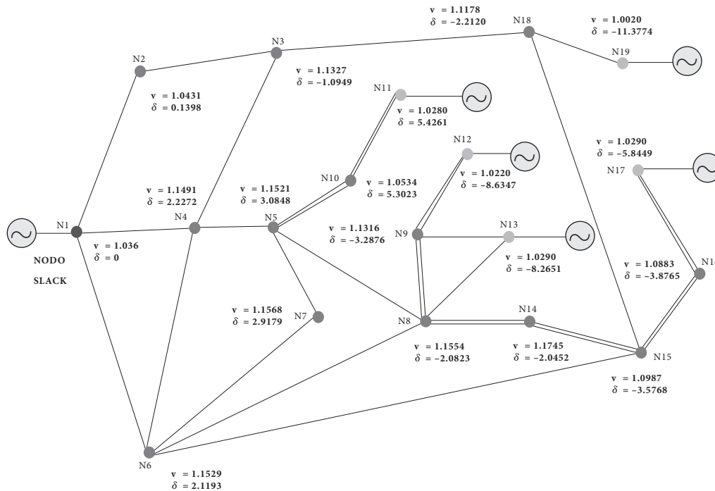
Figura 2.12 Voltajes y ángulos nodales calculados.
