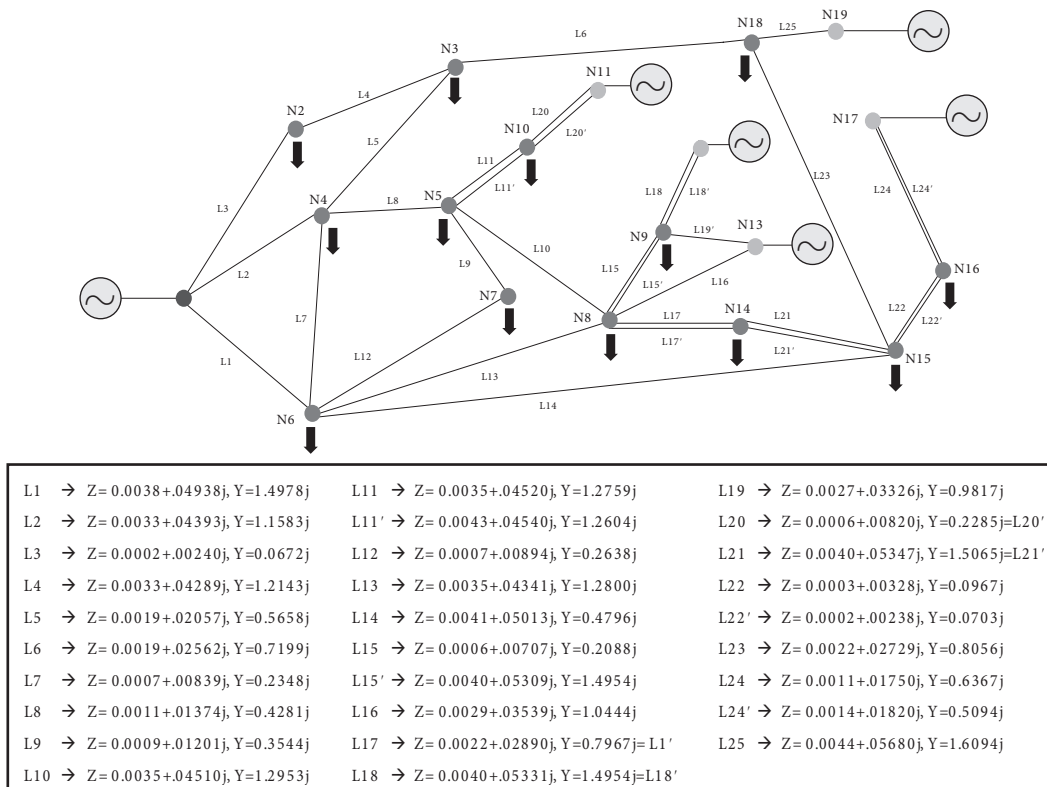
Figura 2.11 Datos de las líneas de la red trifásica.
