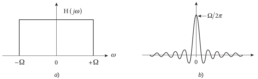
Figura 5.7 Gráficas a) de H(j\omega) y b) de h(t) .
