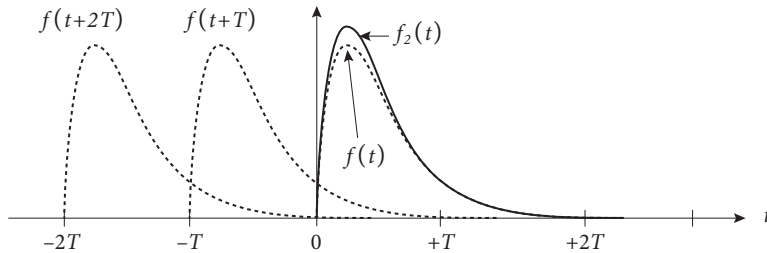
Figura 5.10 Representación f_2(t) como un encimamiento de f(t) y sus desplazamientos.
