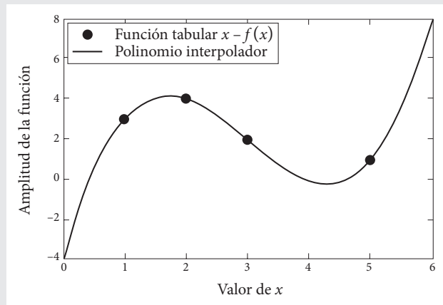
Figura 5.3 Gráfica de la función tabular y del polinomio interpolador P_3(x) .
