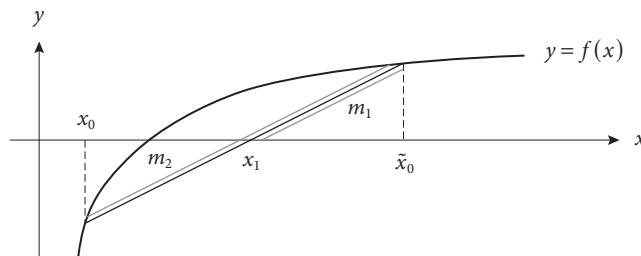
Figura 2.3 Método de la falsa posición.
