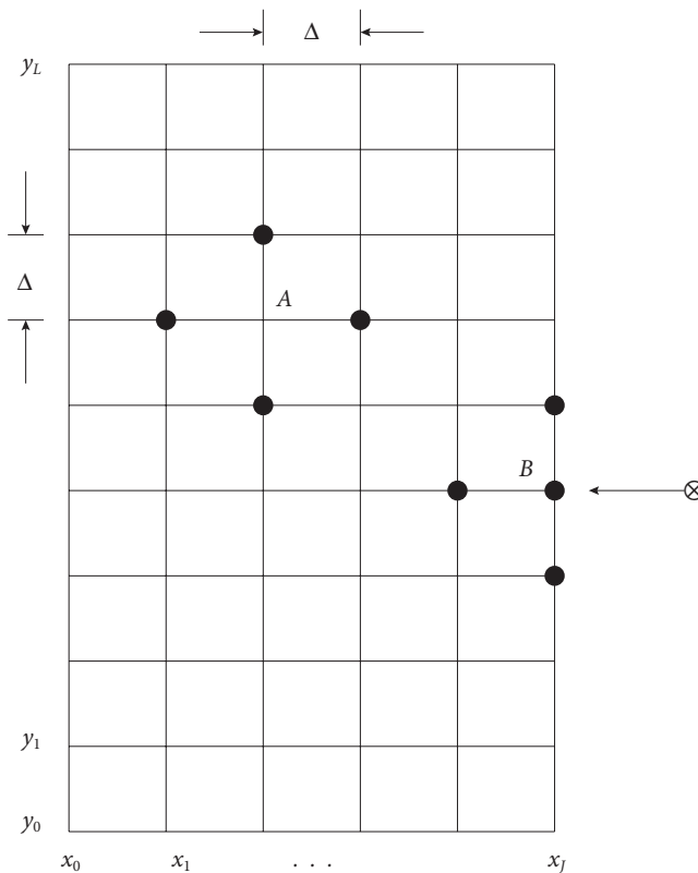
Figura 9.2 Representación en diferencias finitas de una ecuación elíptica de segundo orden sobre una malla bidimensional. Las segundas derivadas en el punto A se evalúan utilizando los valores vecinos a este punto. Las segundas derivadas en el punto B se evalúan utilizando a sus vecinos y a los puntos en la frontera marcados por \otimes .
