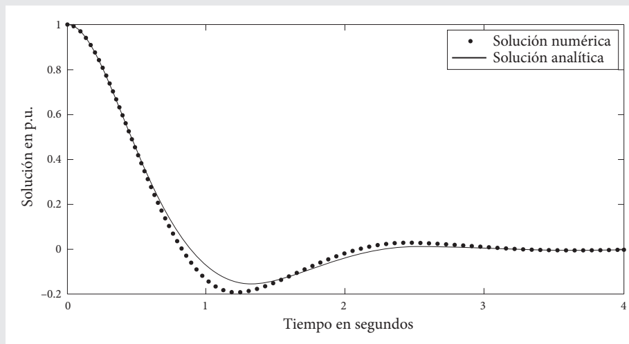
Figura 7.3 Solución numérica con h = 0.05 vs. solución analítica.
