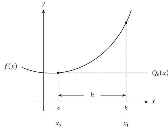
Figura 6.3 Gráfica de la regla rectangular.
