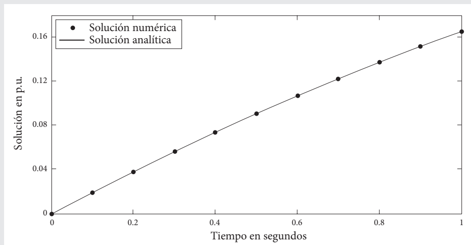
Figura 7.2 Solución numérica vs. solución analítica.
