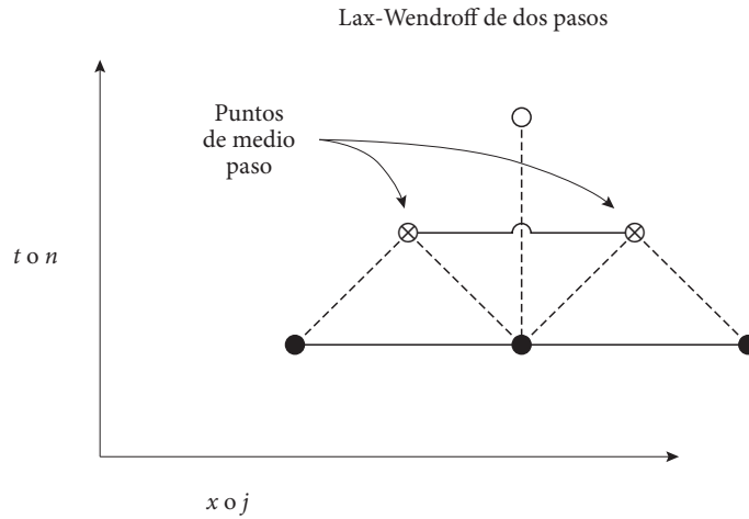
Figura 9.10 Representación del esquema diferenciador Lax-Wendroff de dos pasos. Se calculan dos pasos medios con el método Lax. Éstos, más uno de los puntos originales, producen el punto nuevo a través del salto de rana escalonado.
