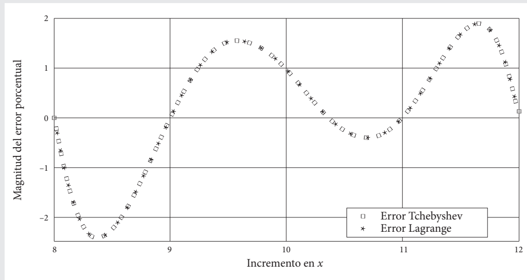
Figura 5.13 Errores porcentuales en el intervalo [8, 12] dado por los dos polinomios interpoladores.
