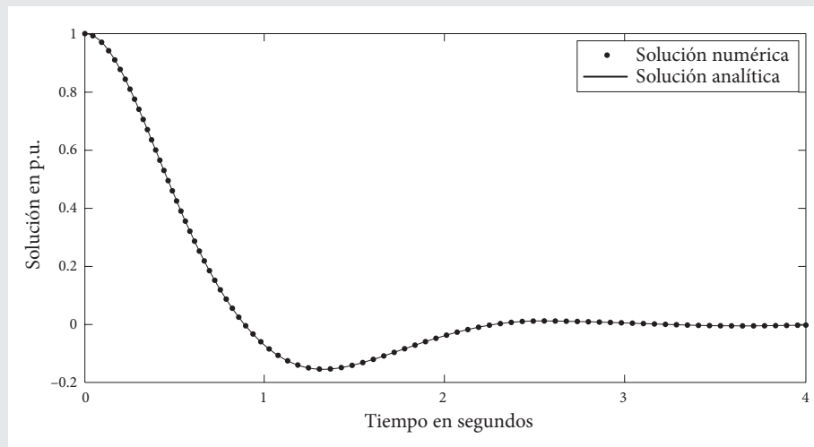
Figura 7.4 Solución numérica con h = 0.01 vs. solución analítica.
