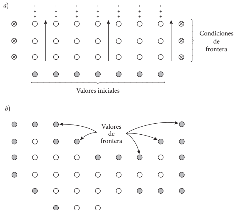
Figura 9.1 Contraste entre un problema de valor inicial a) y el problema de valor de la frontera b). En a) los valores iniciales están dados como una "rebanada de tiempo", apropiada para buscar la solución conforme transcurre éste. En b), los valores de la frontera se especifican alrededor de los bordes de una malla, y se utiliza un proceso iterativo para encontrar los valores de todos los puntos internos (círculos abiertos).
