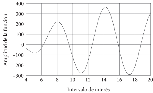
Figura 2.2 Gráfica de la función f(x) .
