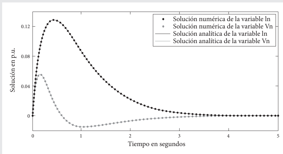
Figura 7.6 Solución numérica del sistema de ecuaciones del ejemplo 7.21, con h = 0.01 .
