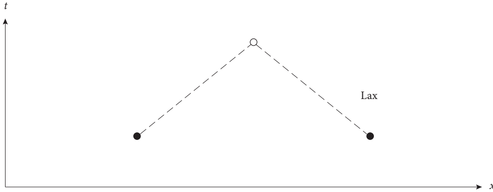
Figura 9.5 Representación del esquema diferenciador Lax. El criterio de estabilidad para este esquema es la condición de Courant .
