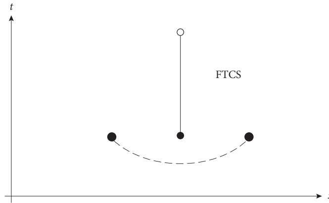
Figura 9.4 Representación del esquema FTCS.
