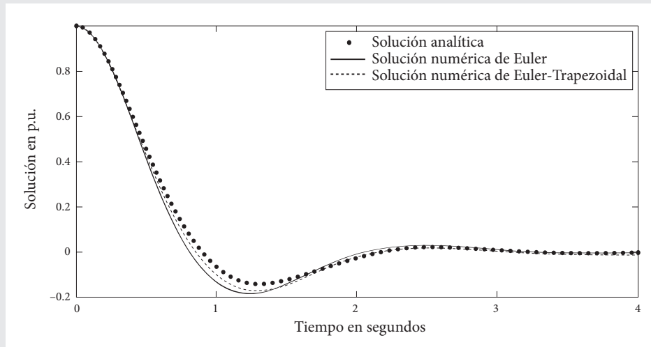
Figura 7.5 Solución numérica con h = 0.05 vs. solución analítica.
