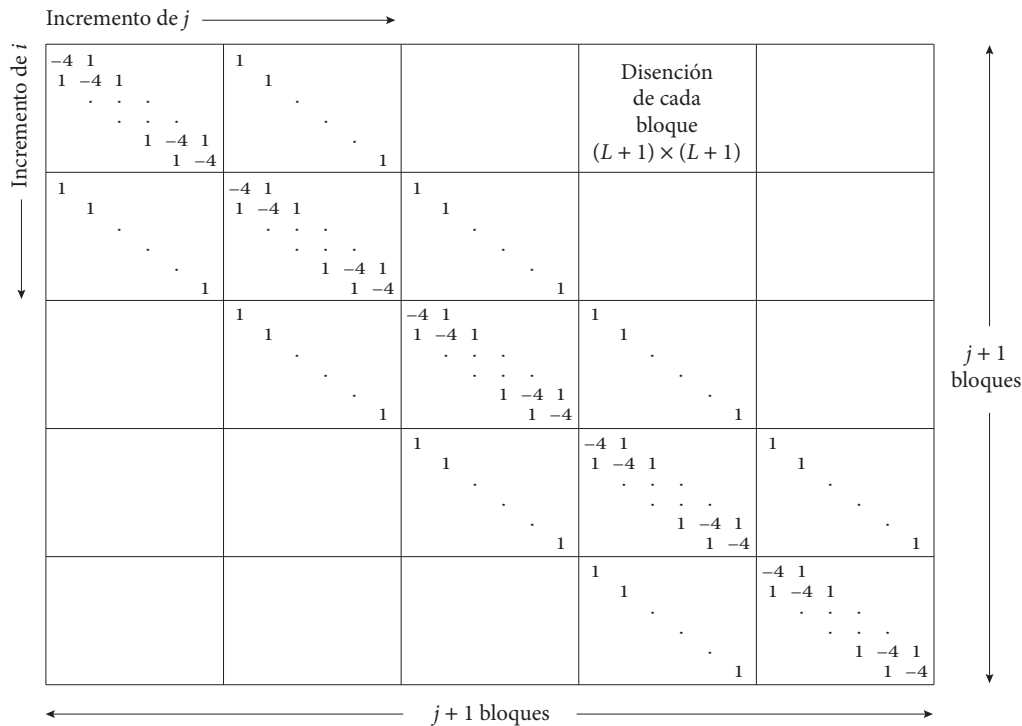
Figura 9.3 Estructura de una matriz que se obtiene de una ecuación elíptica de segundo orden. No todos los elementos son cero. La matriz tiene bloques diagonales que son por sí mismos tridiagonales. Ésta se llama tridiagonal de bloques .
