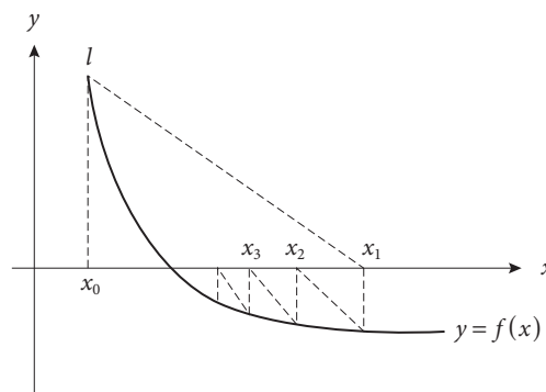
Figura 2.14 Convergencia lenta del método de la falsa posición.
