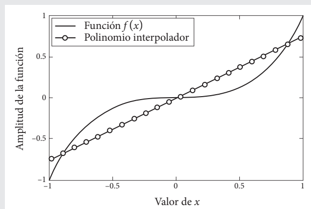
Figura 5.2 Gráfica de la función f(x) y del polinomio interpolador p(x) .
