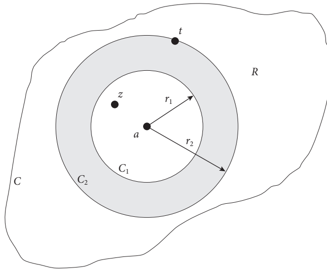
Figura 1.1 Los círculos C_1 y C_2 utilizados en la demostración de la convergencia de la serie de Taylor.
