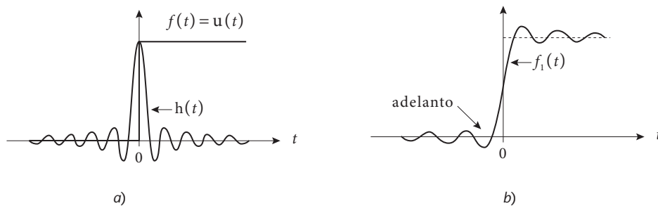
Figura 5.8 Gráficas a) de las funciones f(t) y h(t) y b) de f_1(t) .
