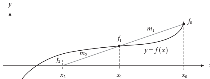
Figura 2.4 Método de la secante.
