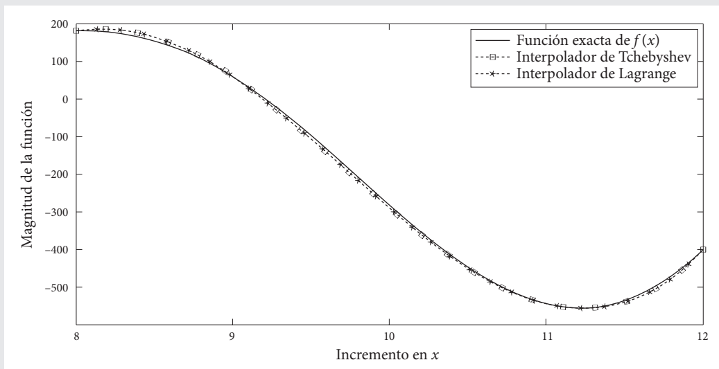
Figura 5.12 Interpoladores de Tchebyshev y de Lagrange con puntos base ortogonales.
