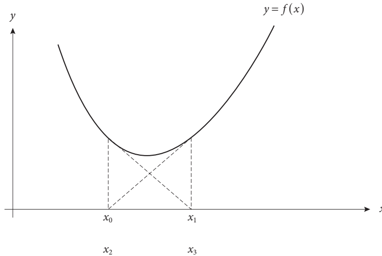
Figura 2.9 Oscilación del método de Newton-Raphson.
