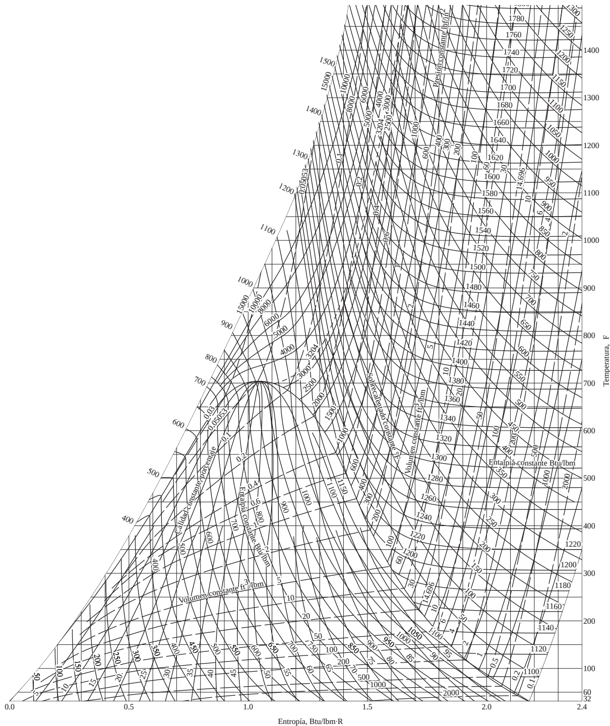
FIGURA A-9E Diagrama T s para el agua.
