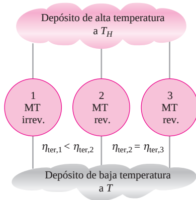
FIGURA 6-40 Principios de Carnot.
