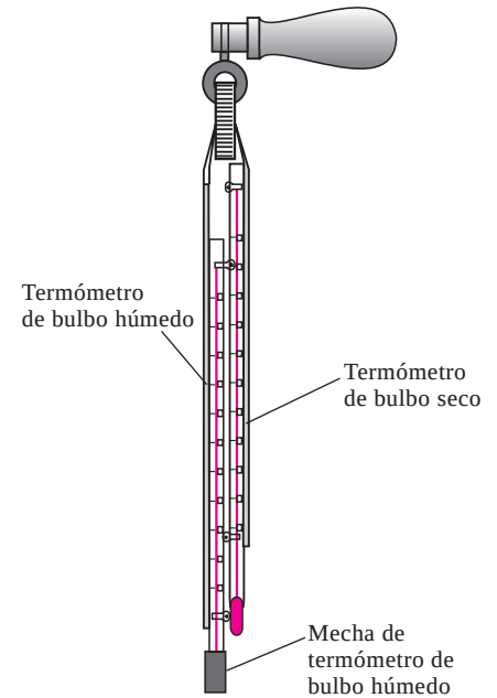
FIGURA 14-13 Psicrómetro giratorio o higrómetro.
