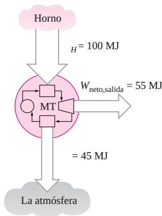
FIGURA 6-14 Incluso las máquinas térmicas más eficientes rechazan casi la mitad de la energía que reciben como calor de desecho.
