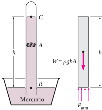
FIGURA 1-51 Barómetro básico.
