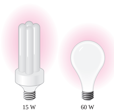
FIGURA 2-55 Una lámpara fluorescente compacta de 15 W provee mucha más luz que un foco incandescente de 60 W.
