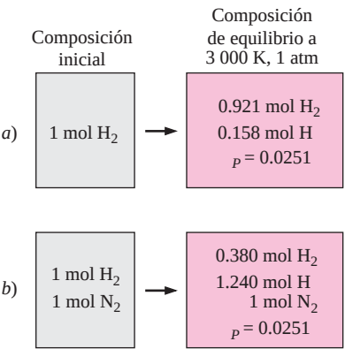
FIGURA 16-10 La presencia de gases inertes no afecta a la constante de equilibrio, sin embargo, afecta la composición de equilibrio.
