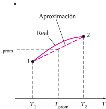
FIGURA 4-26 Para intervalos de temperatura pequeños, se puede suponer que los calores específicos varían en forma lineal con la temperatura.
