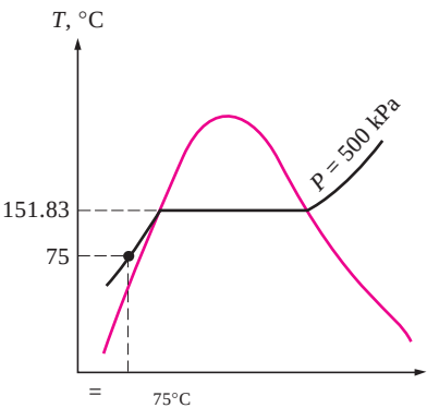
FIGURA 3-44 A P y T dadas, una sustancia pura existirá como un líquido comprimido si T < T_{\text{sat } P} .
