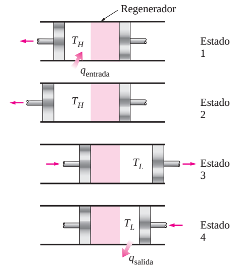
FIGURA 9-27 Ejecución del ciclo Stirling.
